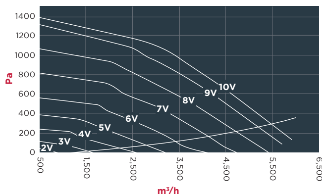
EXTRACT FAN
